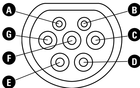
LADEKABEL TYPE 2
